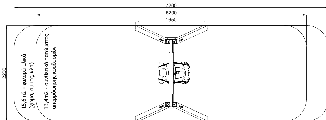
ΚΑΤΟΨΗ ΜΕ ΧΩΡΟ ΠΤΩΣΗΣ
