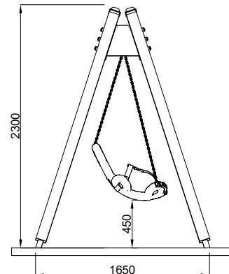
ΠΛΑΓΙΑ ΟΨΗ
