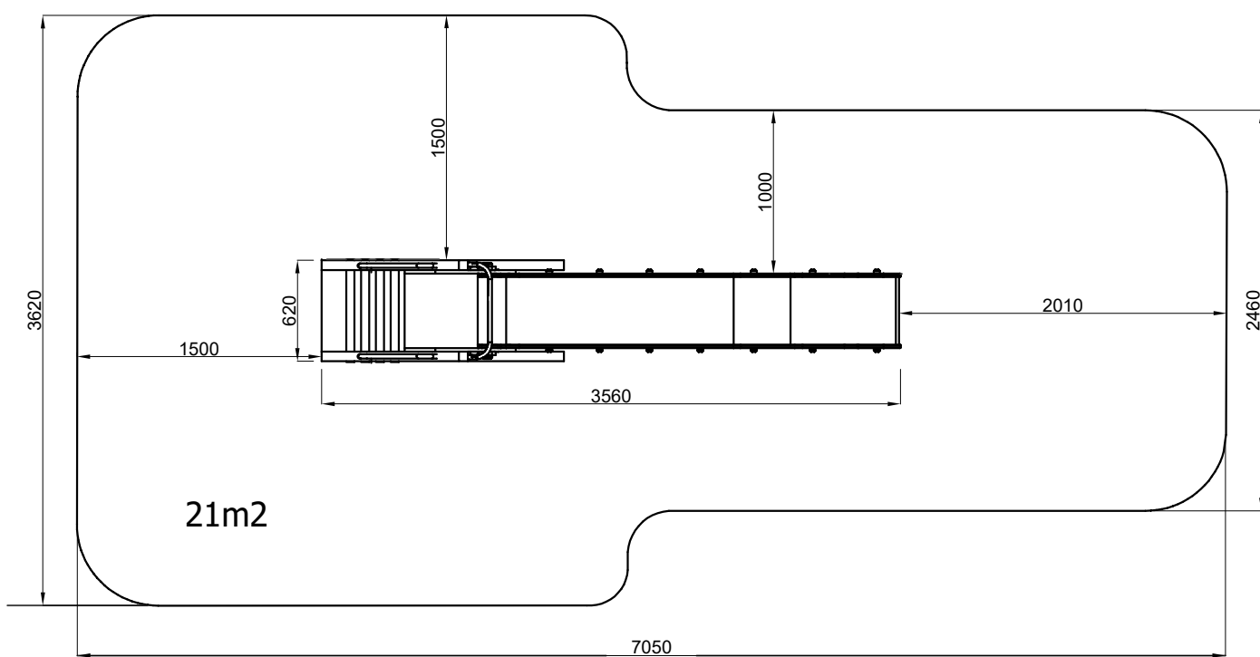
ΚΑΤΟΨΗ ΜΕ ΧΩΡΟ ΠΤΩΣΗΣ
