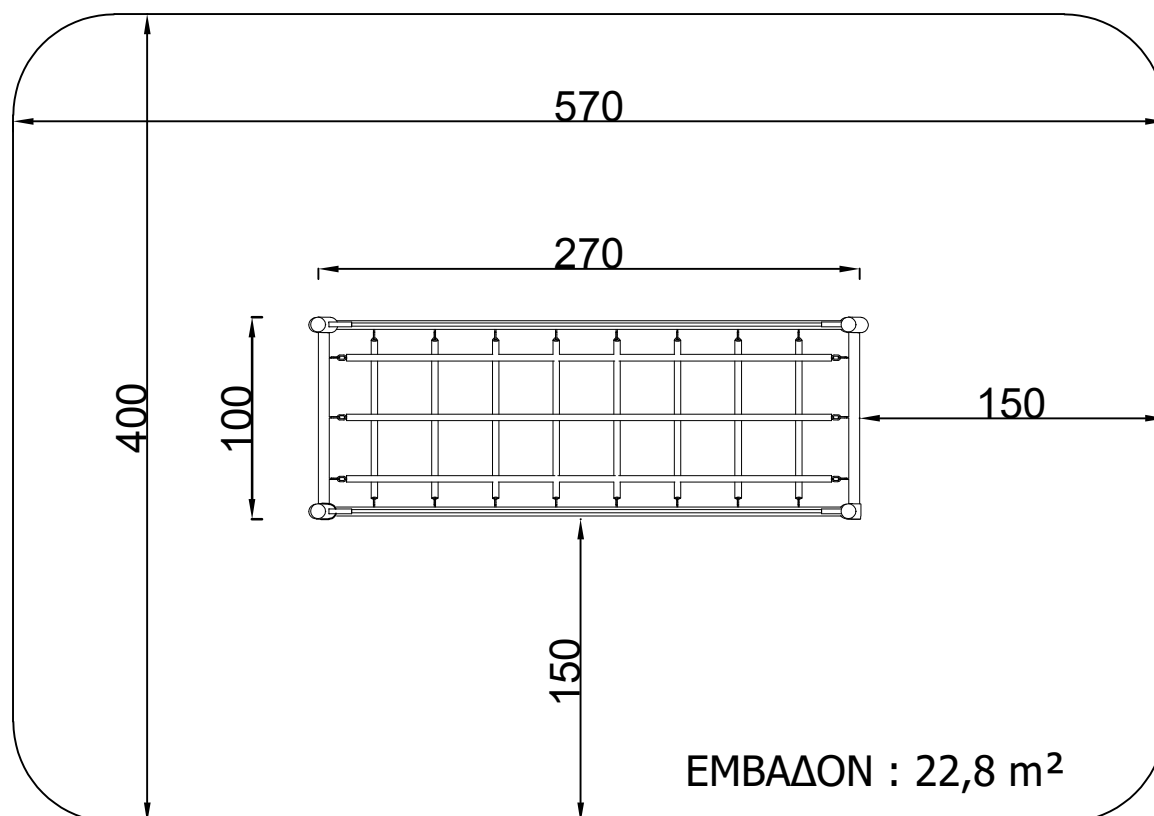
ΚΑΤΟΨΗ
