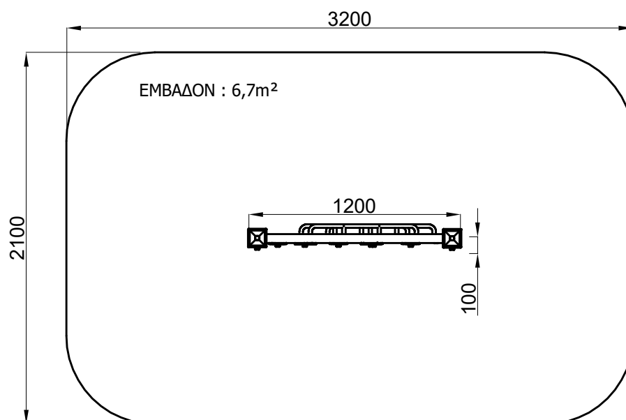
ΚΑΤΟΨΗ ΜΕ ΧΩΡΟ ΠΤΩΣΗΣ
