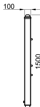
ΠΛΑΓΙΑ ΟΨΗ
