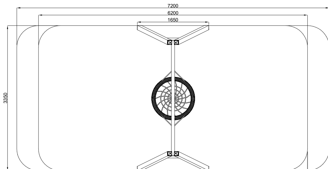
ΚΑΤΟΨΗ ΜΕ ΧΩΡΟ ΠΤΩΣΗΣ
