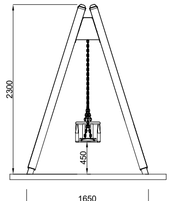
ΠΛΑΓΙΑ ΟΨΗ
