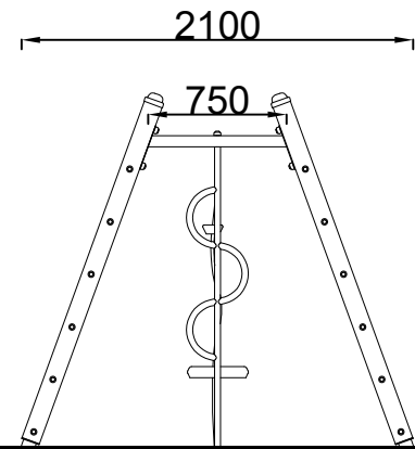
ΠΛΑΓΙΑ ΟΨΗ
