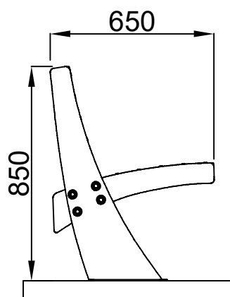
ΠΛΑΓΙΑ ΟΨΗ
