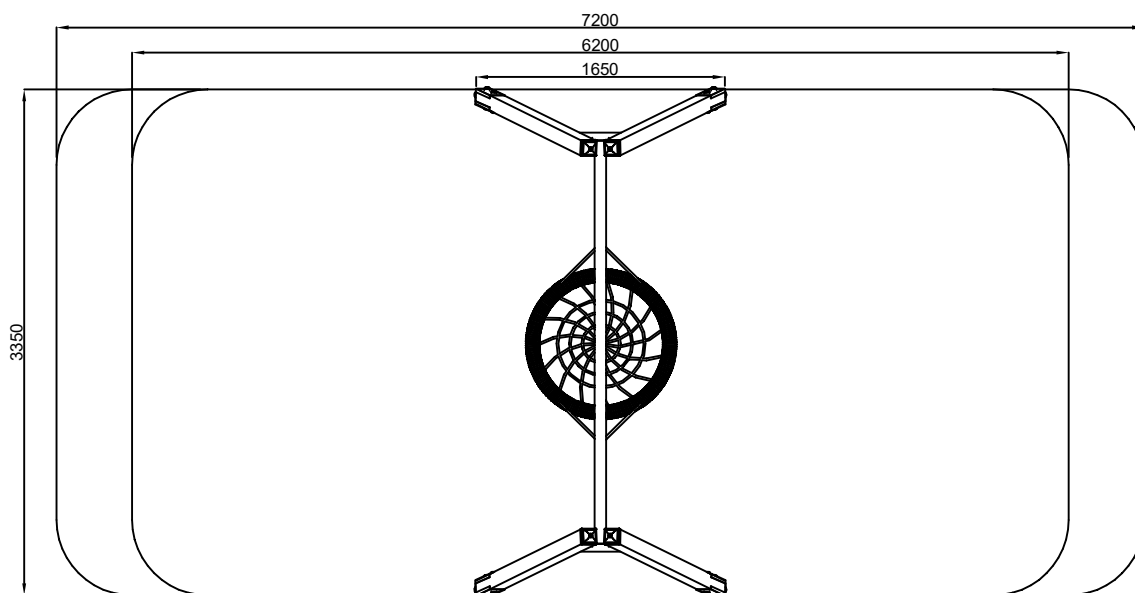
ΚΑΤΟΨΗ ΜΕ ΧΩΡΟ ΠΤΩΣΗΣ
